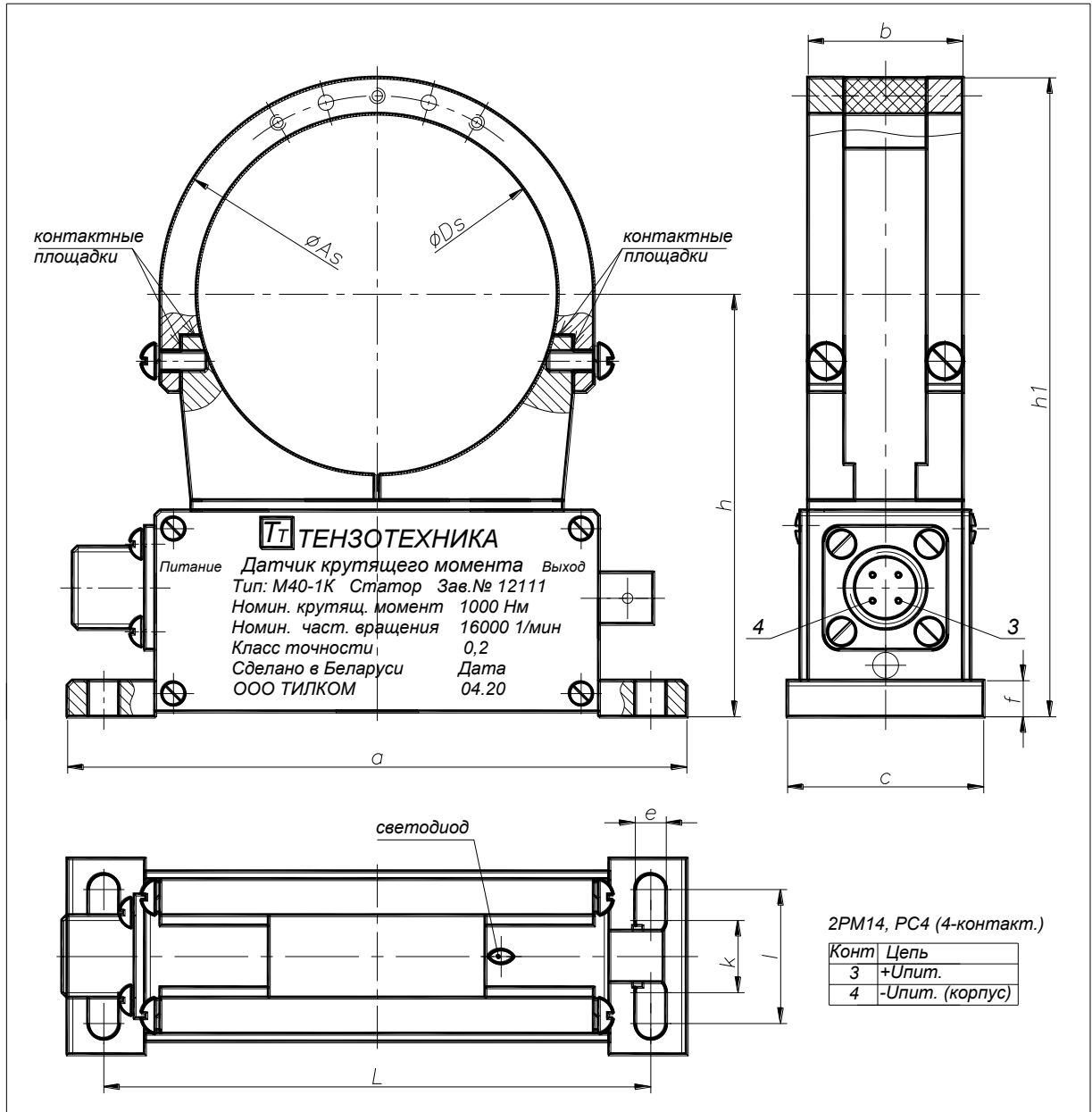
Рисунок 3 - Статор. Габаритные и установочные размеры, мм
