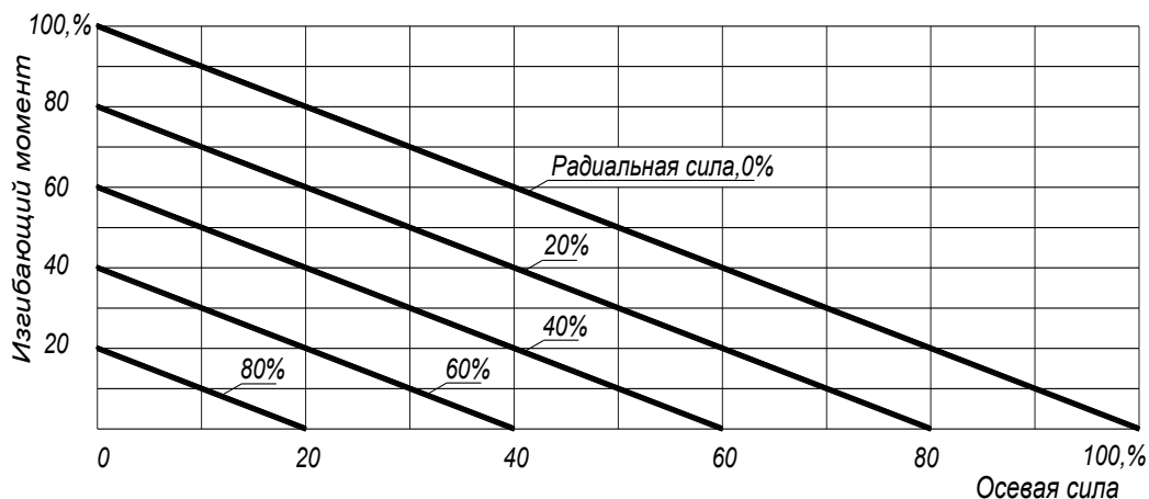
Рисунок 2 - Предельно допустимое сочетание внешних нагрузок
