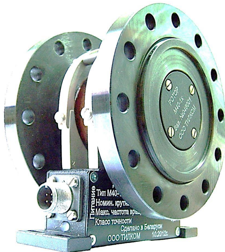
Рисунок 1- Внешний вид датчика крутящего момента М40.
