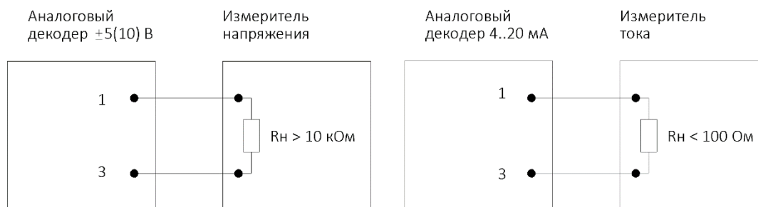
Рисунок 20 - Схема подключения к выходам с аналоговым выходом декодера T24 и блока индикации T42.
