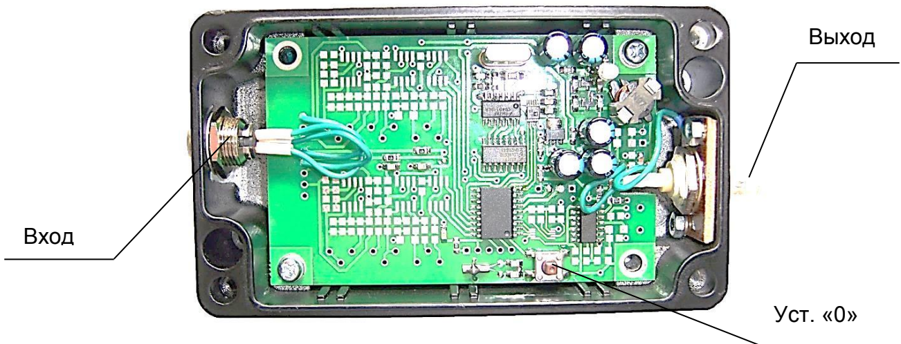
Рисунок 8 - Расположение регулировочных кнопок частотного декодера Т23.
