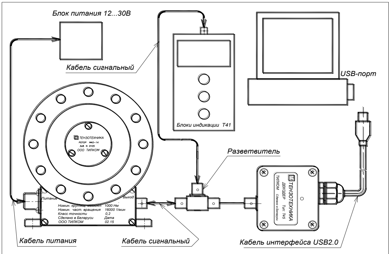
Рисунок 17- Схема подключения датчика к компьютеру и блоку индикации
