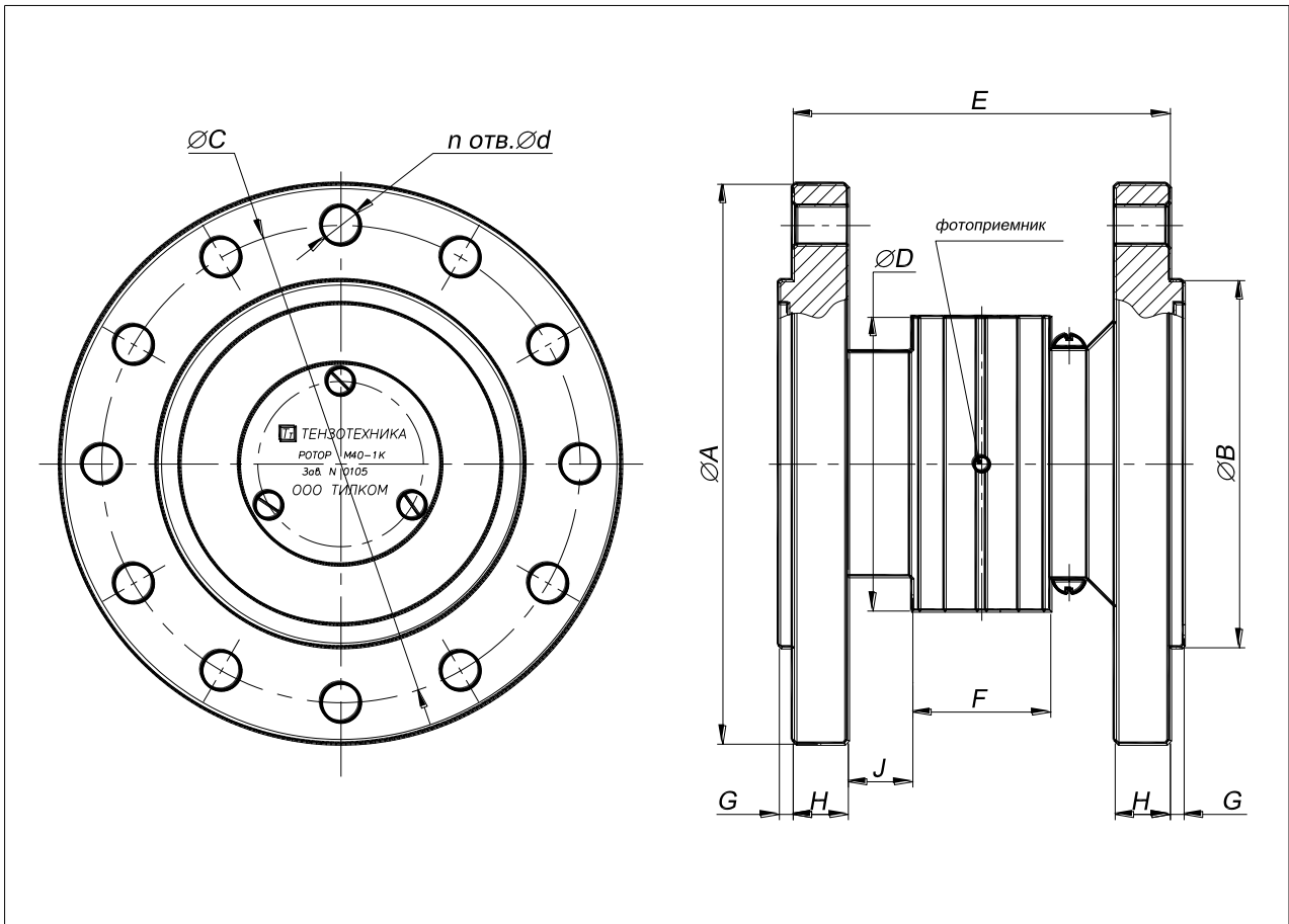
Рисунок 4 - Ротор. Габаритные и установочные размеры, мм.
