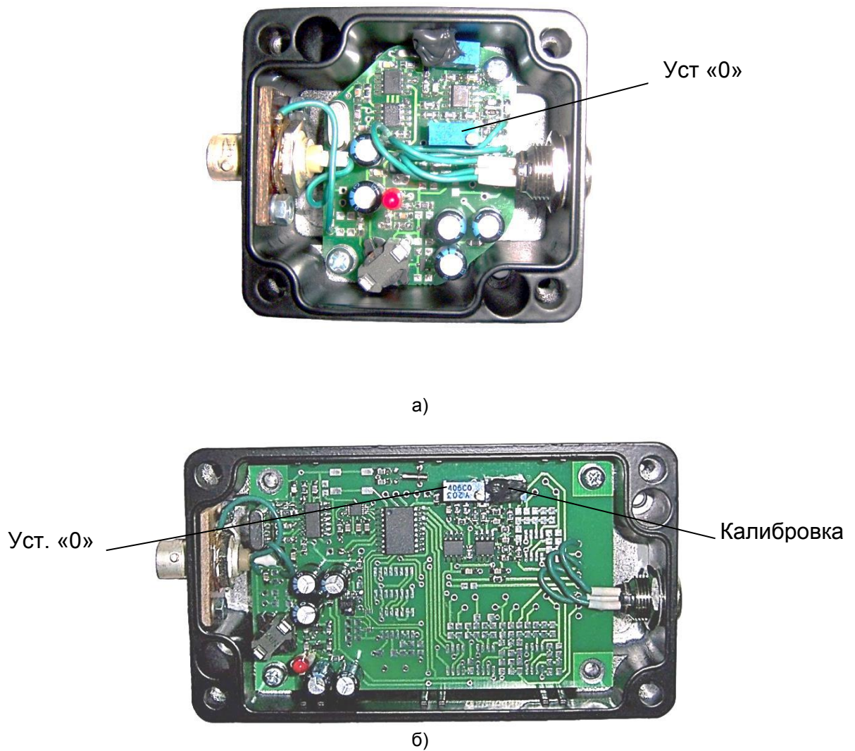
Рисунок 9 - Расположение регулировочных потенциометров аналоговых декодеров Т24(а) и Т24/3(б).
