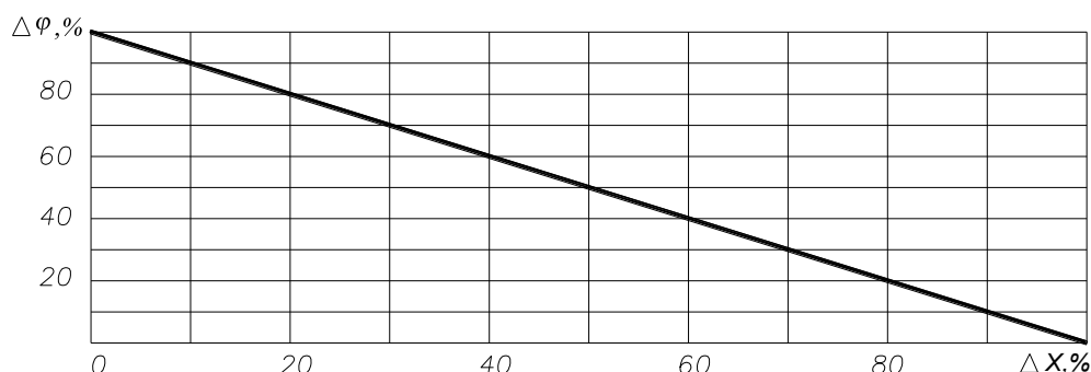
Рисунок 10- Допускаемые сочетания перекося и осевого смещения компенсационных муфт МК
