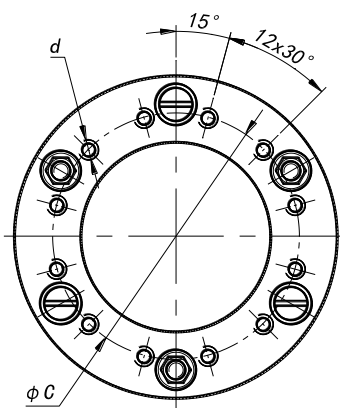
Располож. крепежн. отв. С
