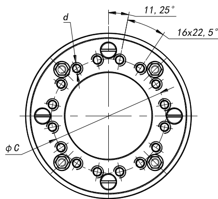
Располож. крепежн. отв. D
