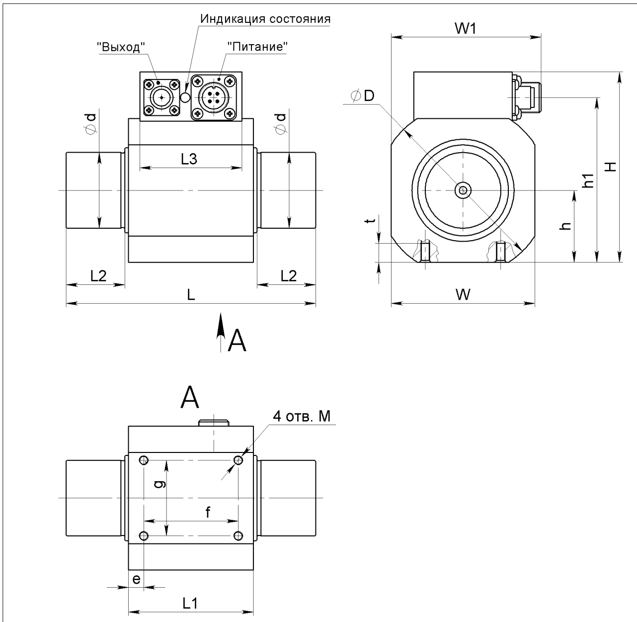
Рис. 4 – Датчики М25-400...М25-5к. Габаритные и установочные размеры, мм
