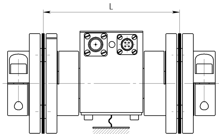
Датчик М25 в сборе с муфтами МВ
