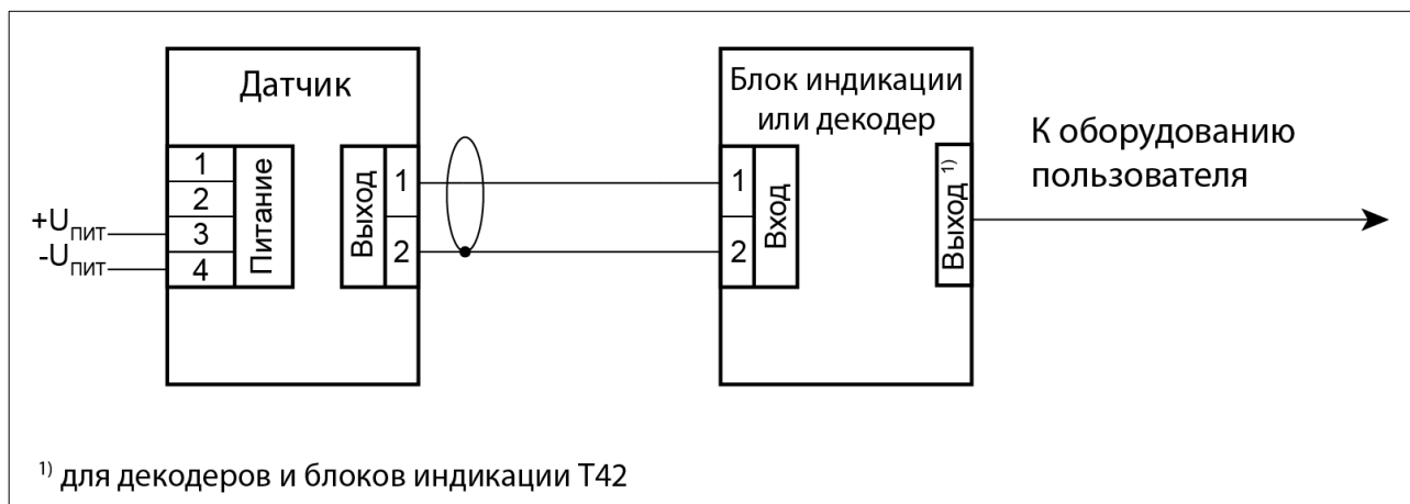
Рис. 9 – Схема подключения датчика М25 к вторичному оборудованию
