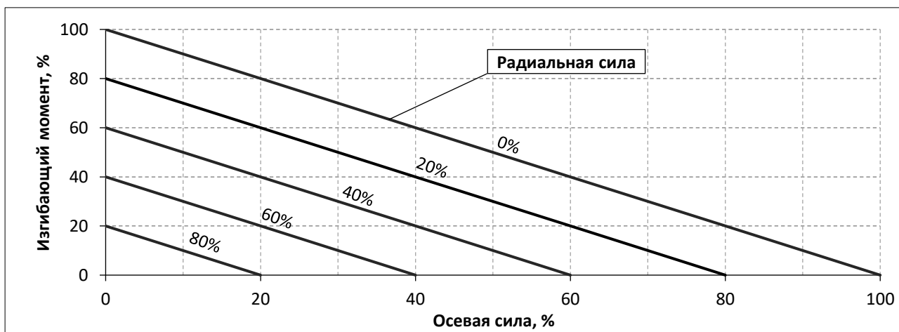
Рис. 2 – Предельно допустимые для датчиков M25 сочетания внешних нагрузок
